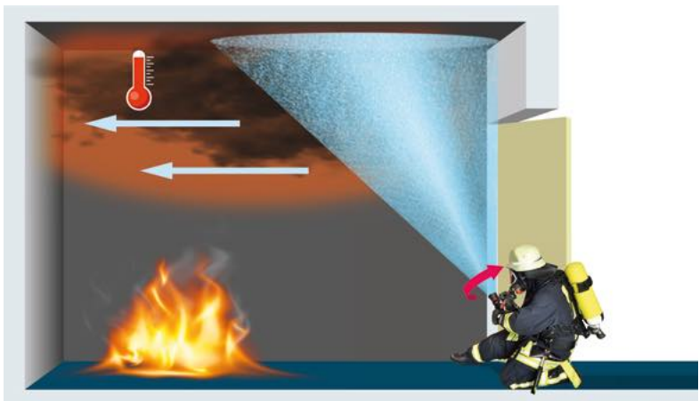
Abb. 32 Raumkühlung
